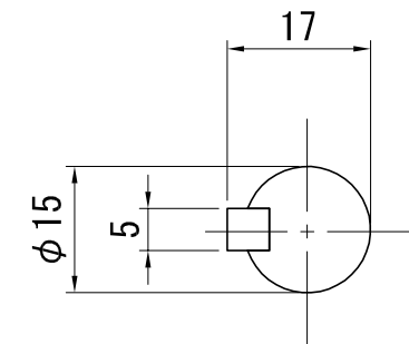
軸端寸法 (1/1)
