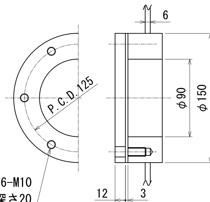
掃除口詳細図
