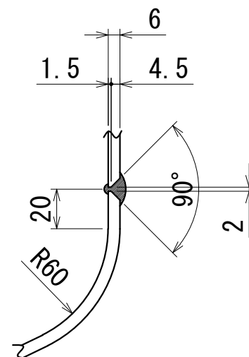
B部詳細図
