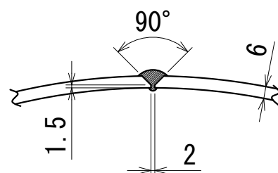
長手継手溶接部詳細図
