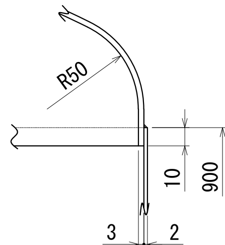
A部周詳細図
