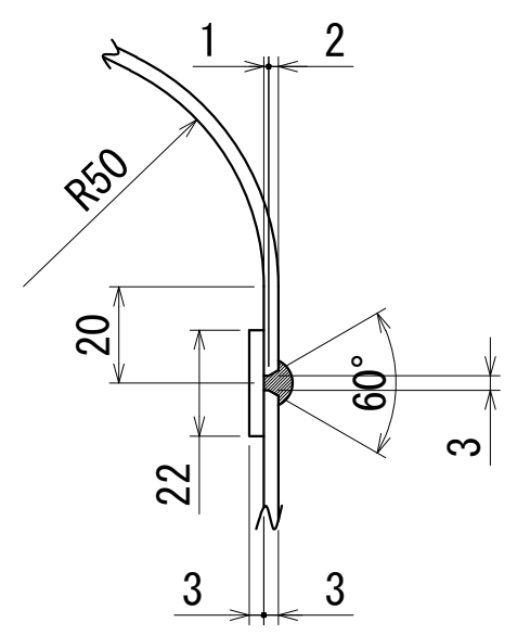
A・B部周継手詳細図
